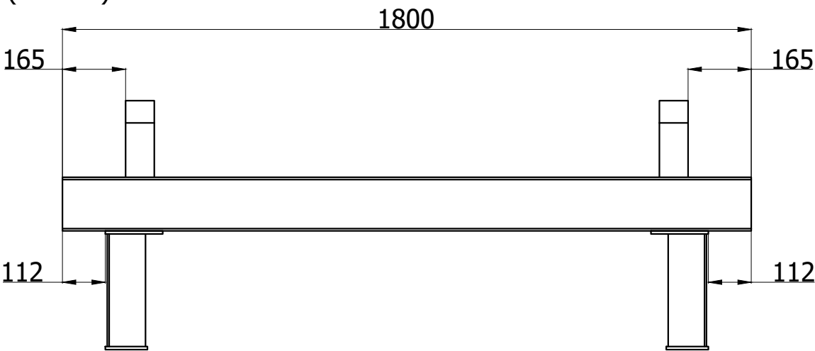
A ( 1 : 4 )
