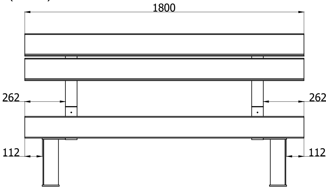
A ( 1 : 4 )
