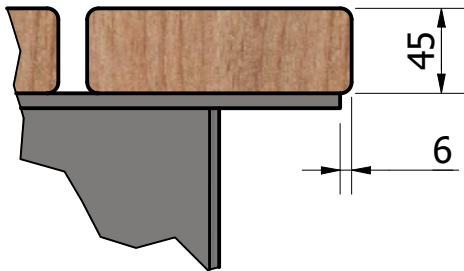
A ( 1 : 4 )
