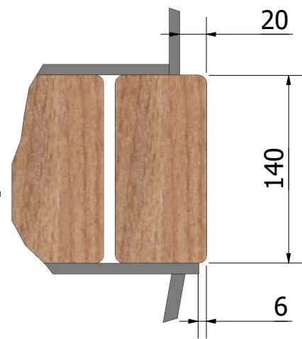
A ( 1 : 4 )
