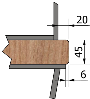
A ( 1 : 4 )
