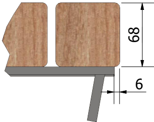
A ( 1 : 4 )
