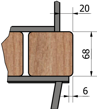
A ( 1 : 3 )
