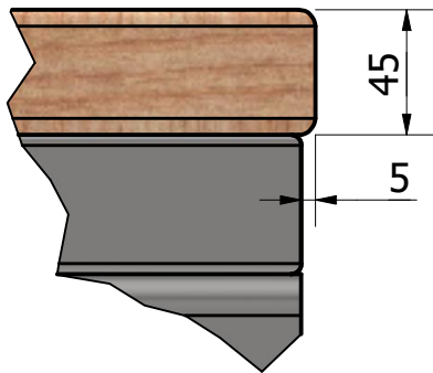
A ( 1 : 3 )
