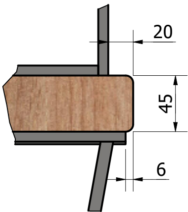
A ( 1 : 3 )
