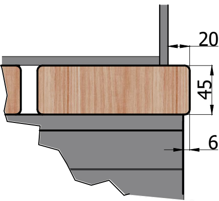
A ( 1 : 4 )
