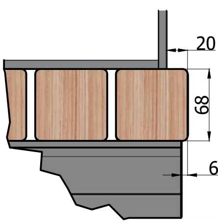
A ( 1 : 4 )
