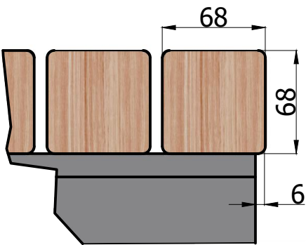
A ( 1 : 4 )
